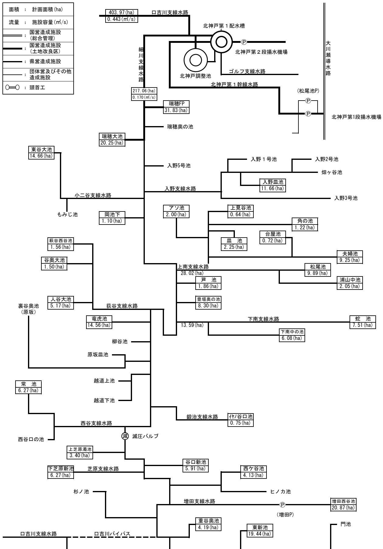
配水ブロック図(細川支線水路)
