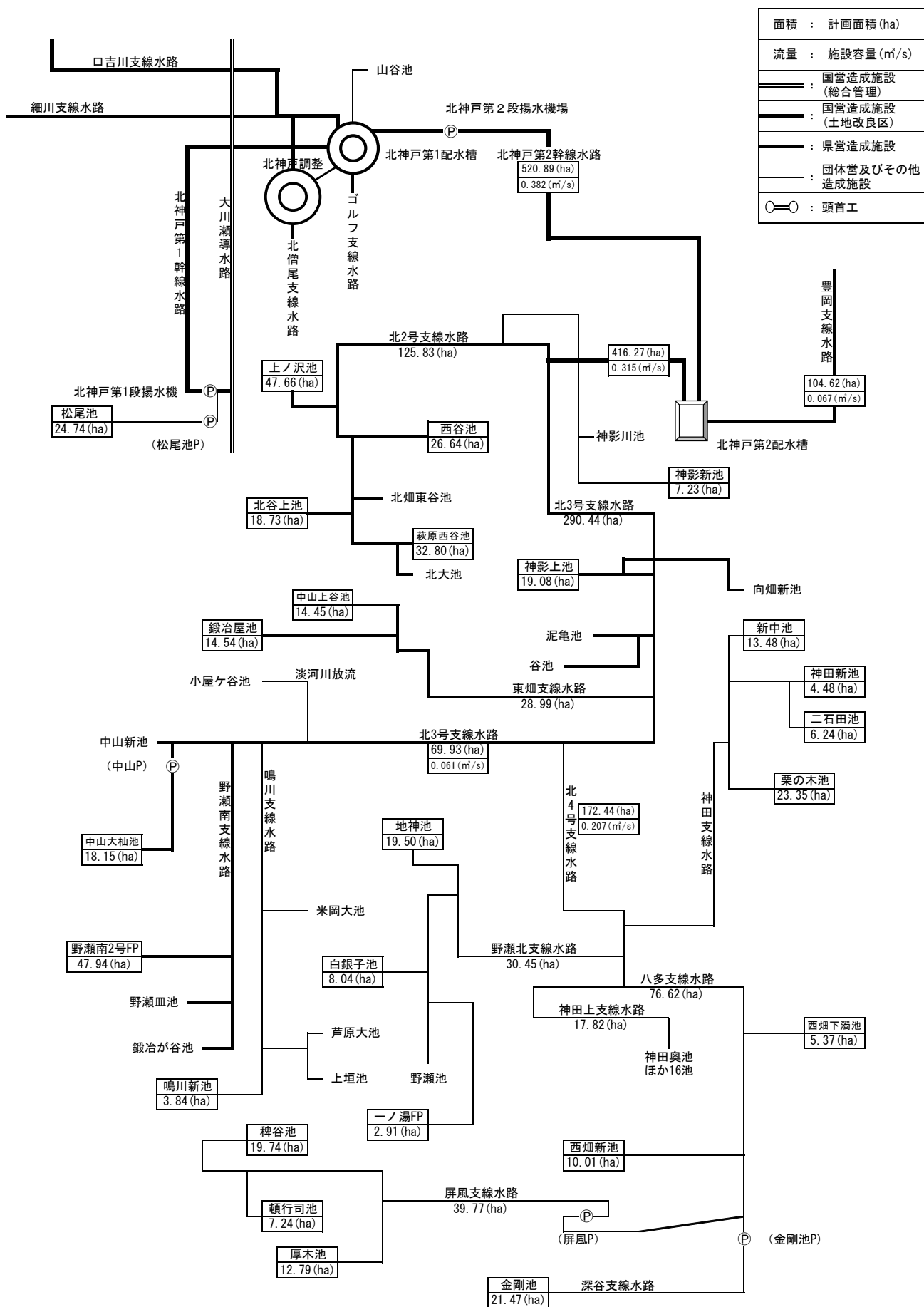
配水ブロック図（北神戸第2幹線水路）
