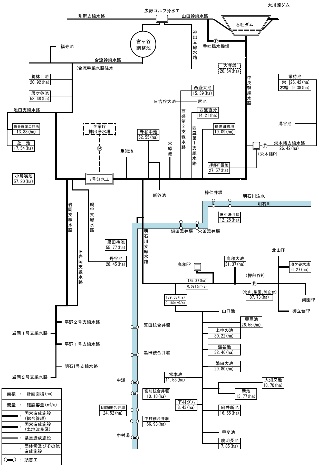
配水ブロック図（中央幹線水路）
