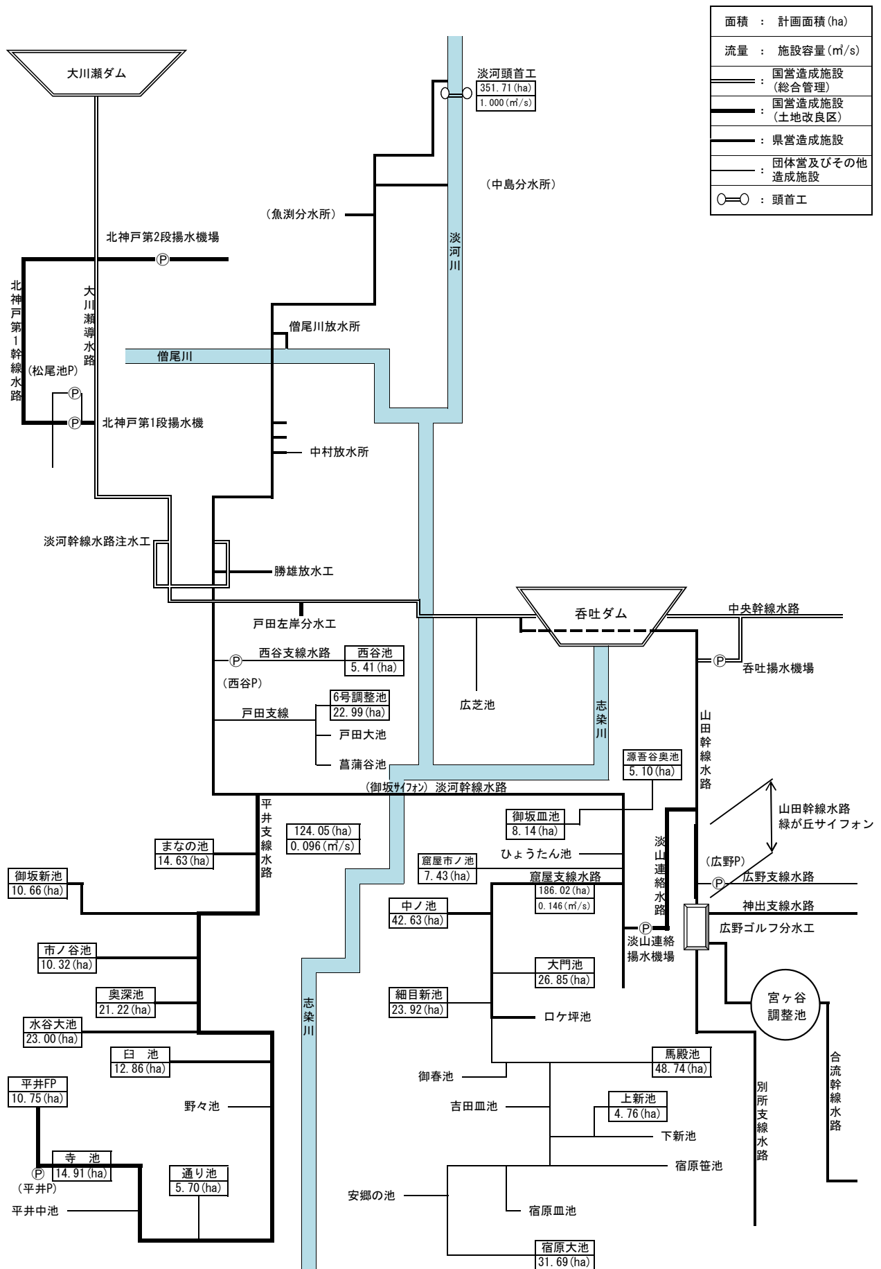
配水ブロック図（淡河幹線水路）
