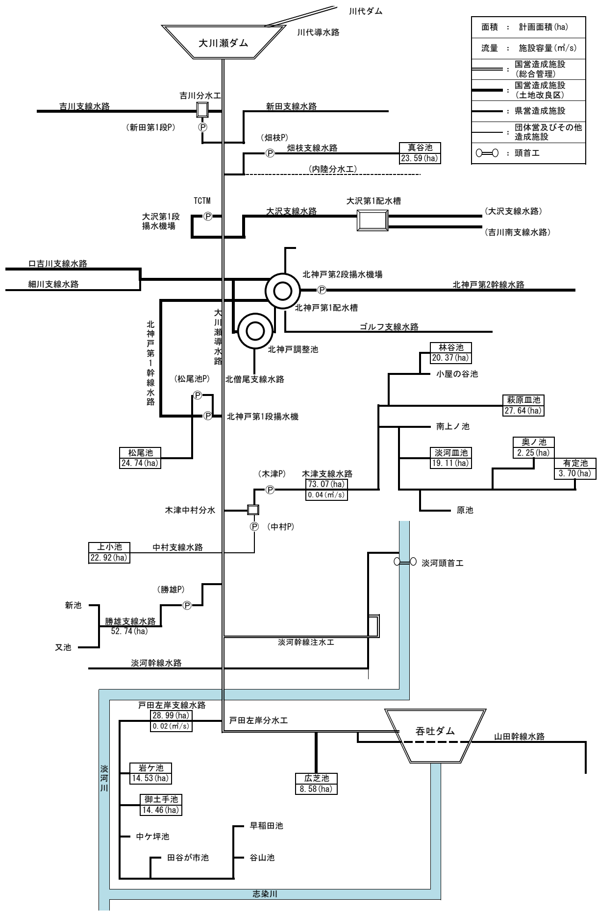
配水ブロック図（大川瀬導水路）
