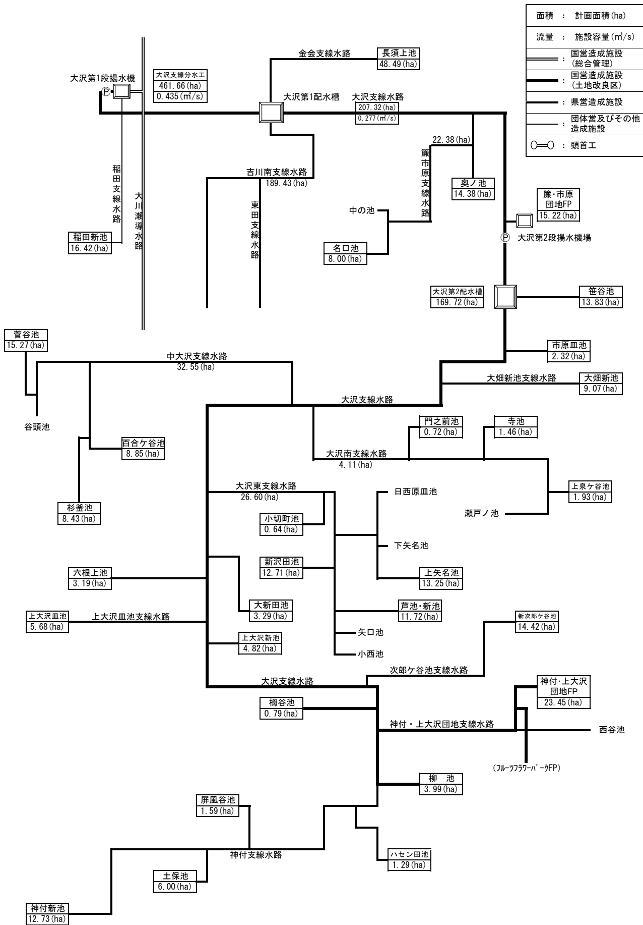
配水ブロック図（大沢支線水路）
