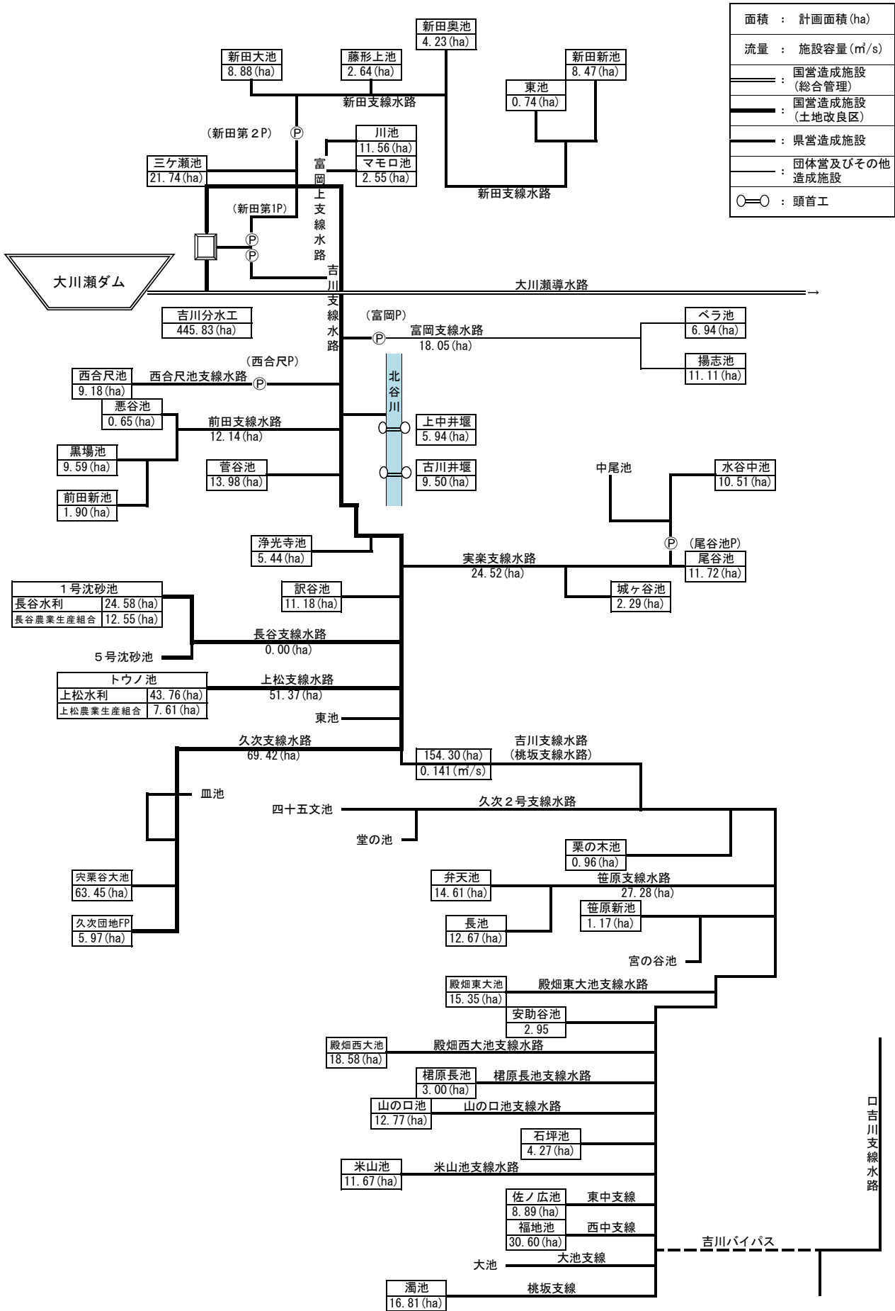
配水ブロック図（吉川支線水路）
